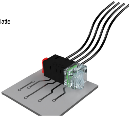
Abb. 1: Direktsteck- Technologie (Steckverbindersockel entfällt)
