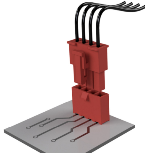
Abb. 2: Herkömmliche Steckverbinderlösung mit Gegenstecker
